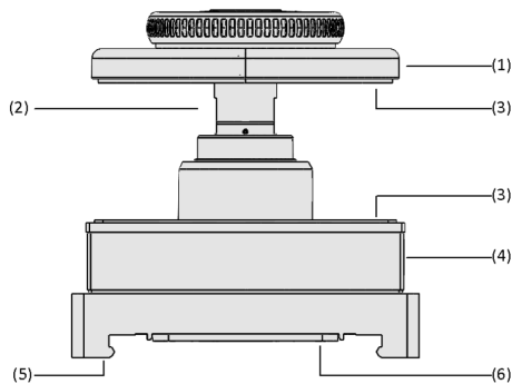
Design del sistema Bloccaggi meccanici VCMC-S4-QUICK
